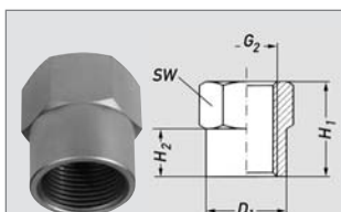
Nátrubek
