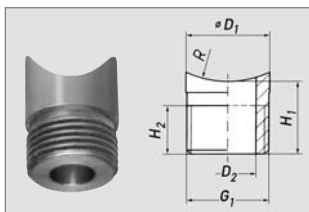
Závitový návarek s rádiusem (R = 10/13/16/20/25 nebo 31 mm)
