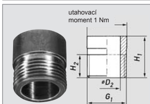
Závitový návarek
