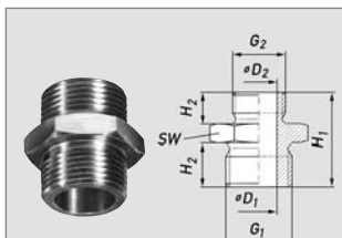
Závitová přechodka
